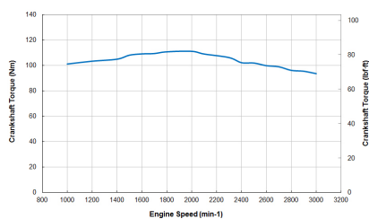
Krouticí moment
