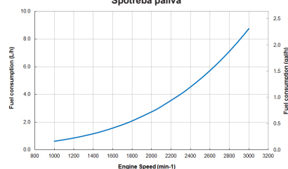
Spotřeba paliva
